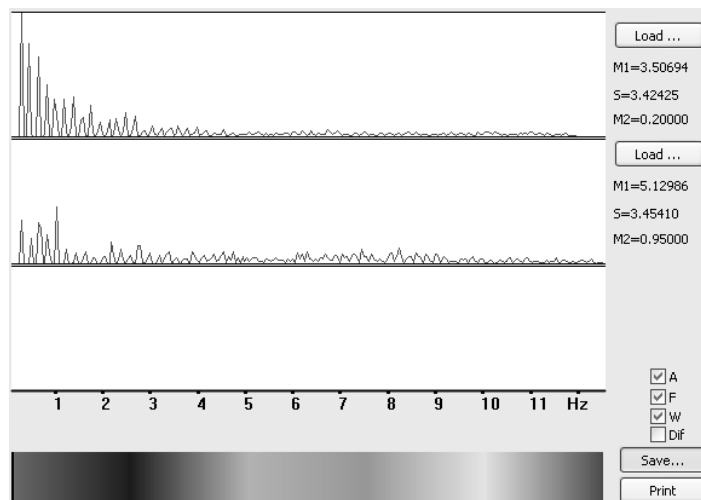
Рис. 4. Спектр сигнала виброизображения (программное окно) человека в нормальном состоянии на верхнем графике и в тревожном состоянии на нижнем графике.
