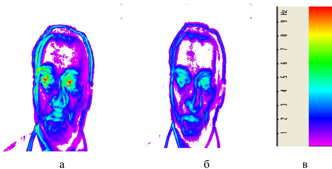
Рис.1. Амплитудное (а), частотное (б) виброизображение человека, псевдоцветовая шкала (в).
