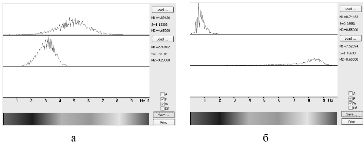
Рис. 3. Гистограмма (программное окно) распределения частоты вибраций для человека в нормальном психофизиологическом состоянии (а) и в экстремальном психофизиологическом состоянии (б), верхний график характеризует усталость, нижний график характеризует ярость.
