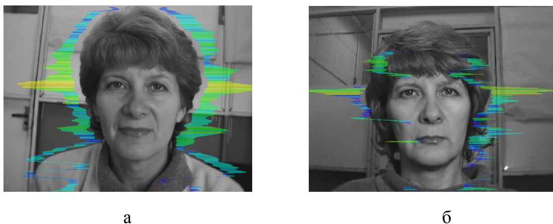
Рис. 2. Внешнее виброизображение человека в спокойном состоянии (а) и в состоянии стресса (б).
